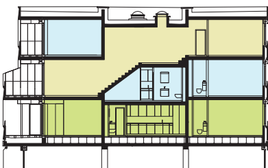
Querschnitt durch die Aufstockung (7.-9. Obergeschoss).
