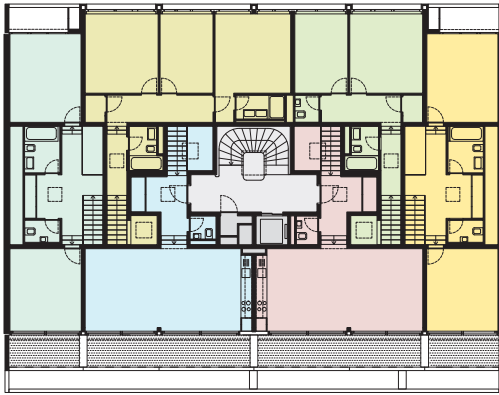
9. Obergeschoss (Ausschnitt).
