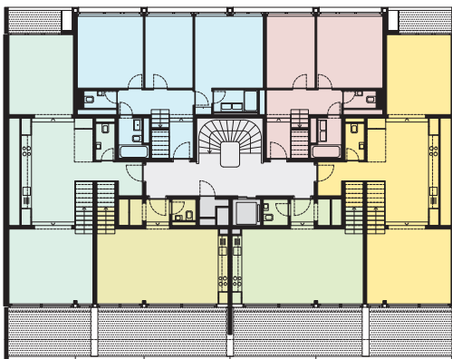
8. Obergeschoss (Ausschnitt).
